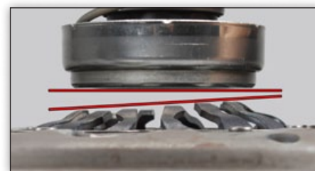
Fig. 4: Incorrecte montage
