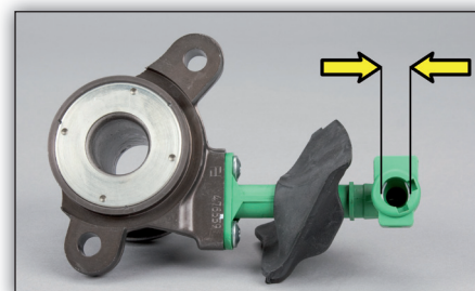
Fig. 4: LuK hydraulisch scharnierstuk 510 0137 10 hydraulische aansluiting 12,2 mm
