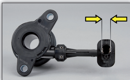
Fig. 1: LuK hydraulisch scharnierstuk 510 0090 10 hydraulische aansluiting 12,2 mm
