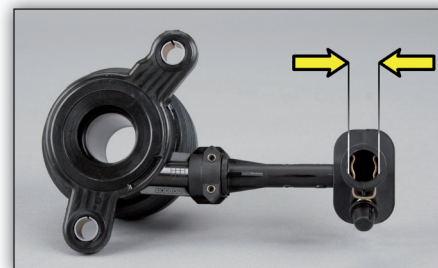
Fig. 2: LuK hydraulisch scharnierstuk 510 0097 10 hydraulische aansluiting 13,3 mm
