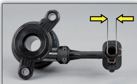
Fig. 3: LuK hydraulisch scharnierstuk 510 0098 10 hydraulische aansluiting 11,7 mm
