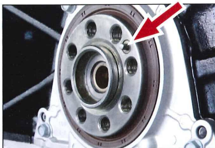
Figuur 1: Krukas centreer pin.
